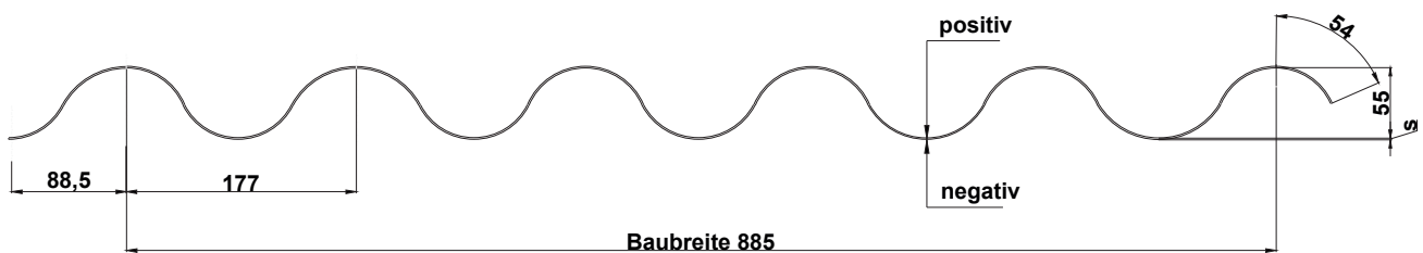
Einbausituation Dach & Wand Baubreite 885mm
