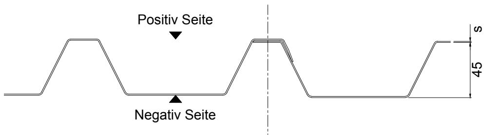
Einbausituation Dach Breite 900mm
