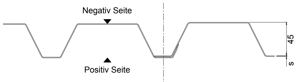
Einbausituation Wand Breite 900mm
