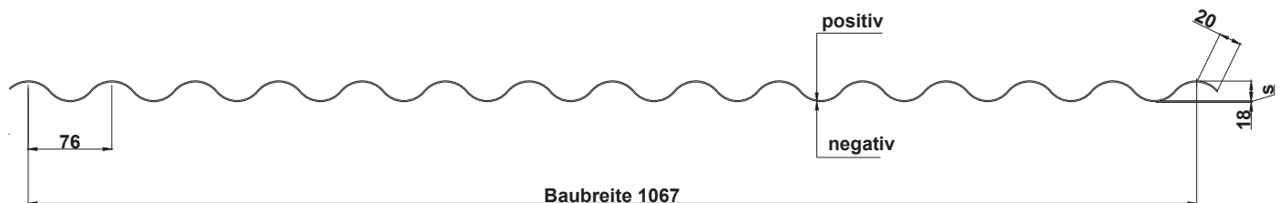
Einbausituation Wand Baubreite 1067mm
