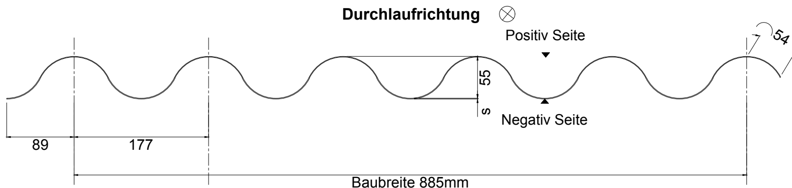
Einbausituation Dach & Wand Baubreite 885mm
