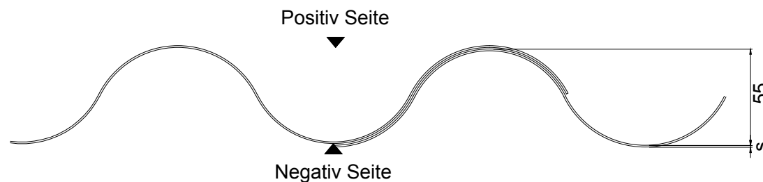
Einbausituation Dach & Wand Baubreite 885mm
