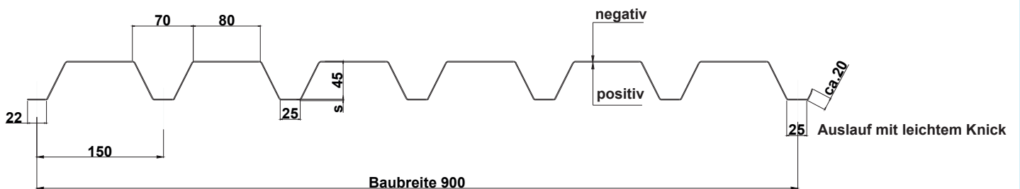
Einbausituation Dach
