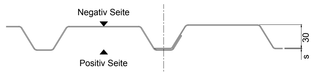
Einbausituation Wand Breite 1071mm
