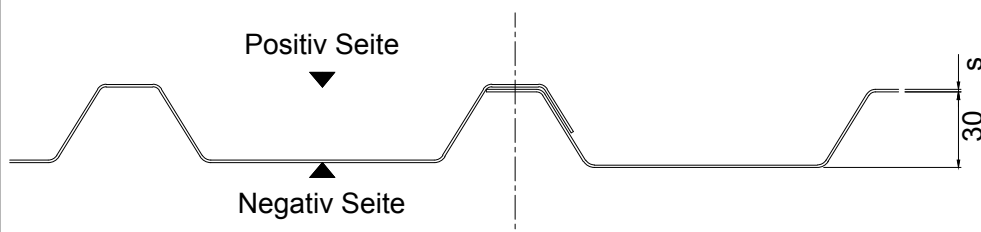
Einbausituation Dach Breite 1071mm
