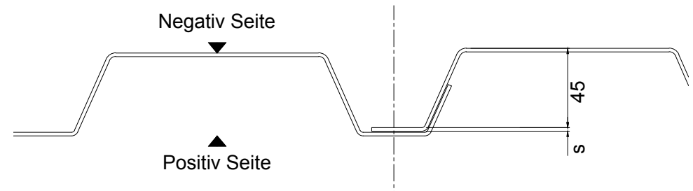
Einbausituation Wand Breite 1000mm
