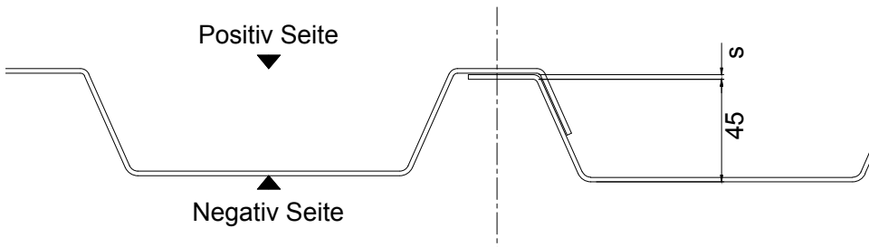
Einbausituation Dach Breite 1000mm
